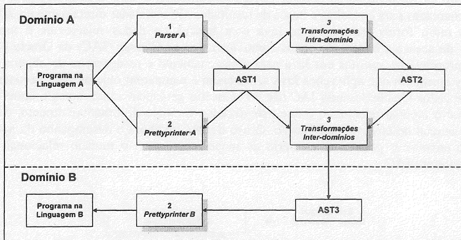
FIGURA 3 - PARTES DE UM DOMÍNIO NO DRACO-PUC
